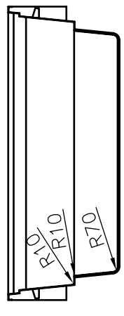
B-B
