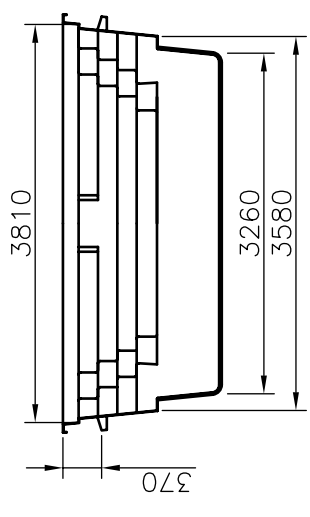
C-C
