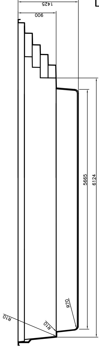
Doorsnede A-A
